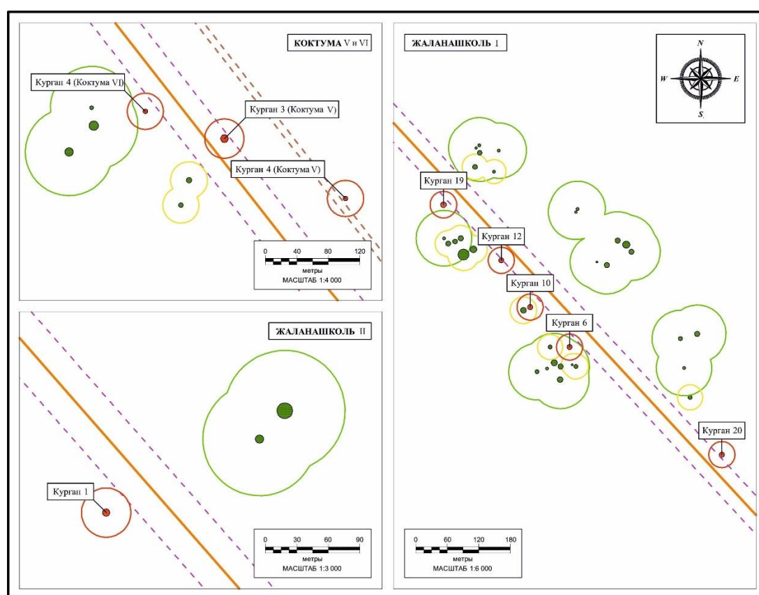
Рис. 4. Схема расположения исследованных курганов в могильниках близ сел Коктума и Жаланашколь
